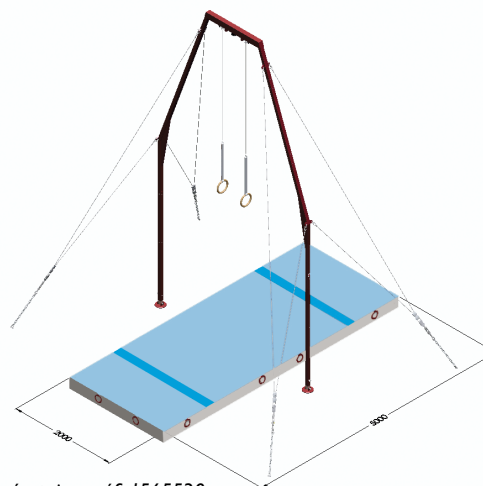
Jeu de tapis de réception : réf. 1565530
